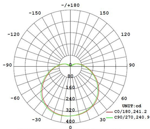
diagrama de distribución de la intensidad luminosa
